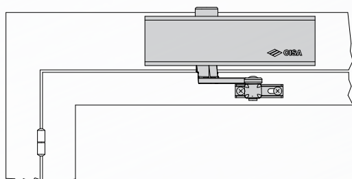
Montaggio lato opposto cerniere, porte con apertura verso esterno
